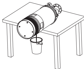
Рис. 9 Слив масла
