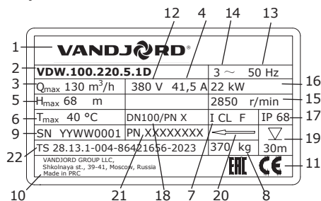
Рис. 2 Фирменная табличка
